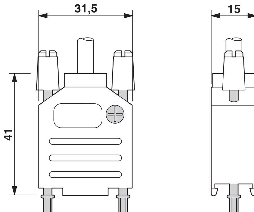
Dessin coté
