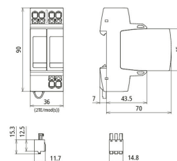
Dimensioni DG MP TT 2P ACI 385 FM
