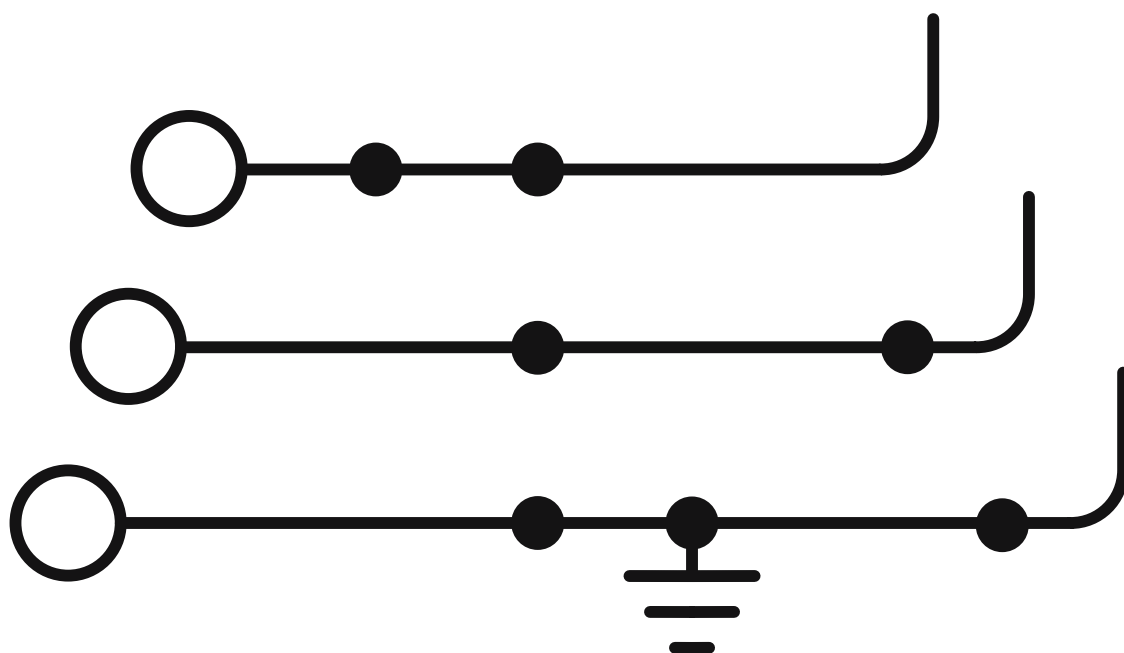
Diagrama eléctrico
