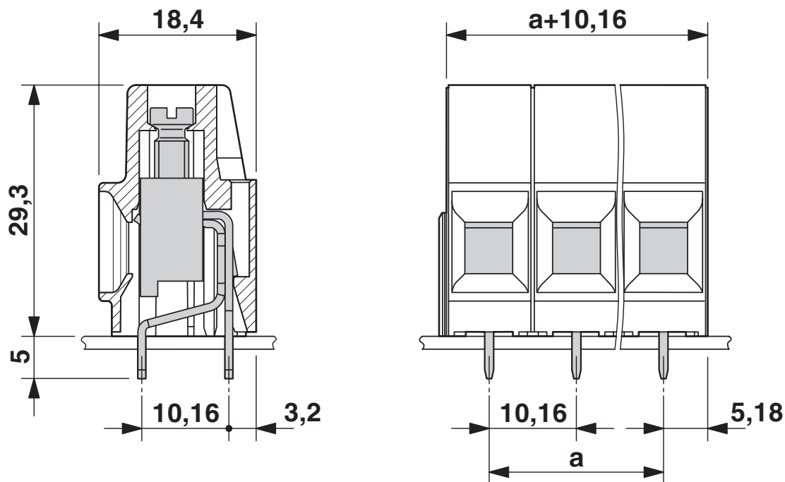
Maßzeichnung
