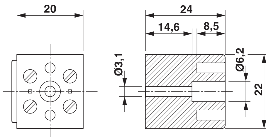
Dessin coté
