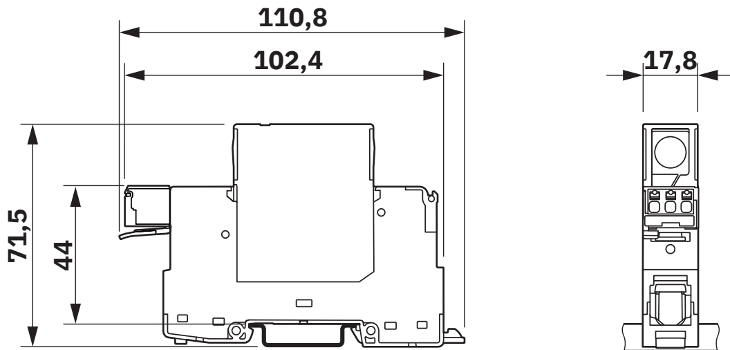
Dessin coté
