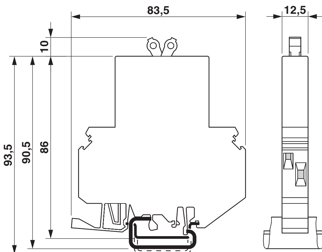
Dessin coté
