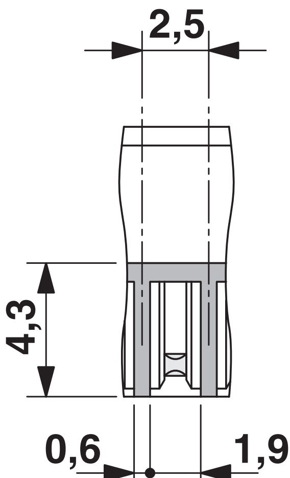
Dessin coté
