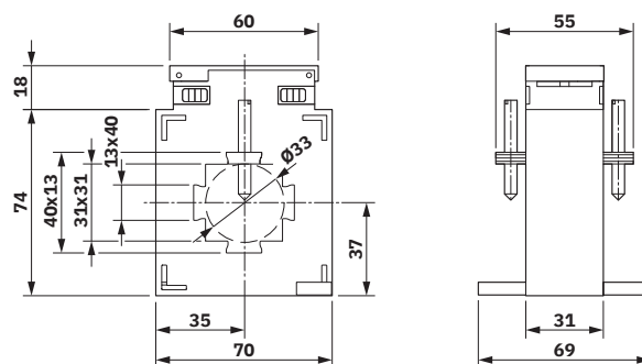
Dessin coté
