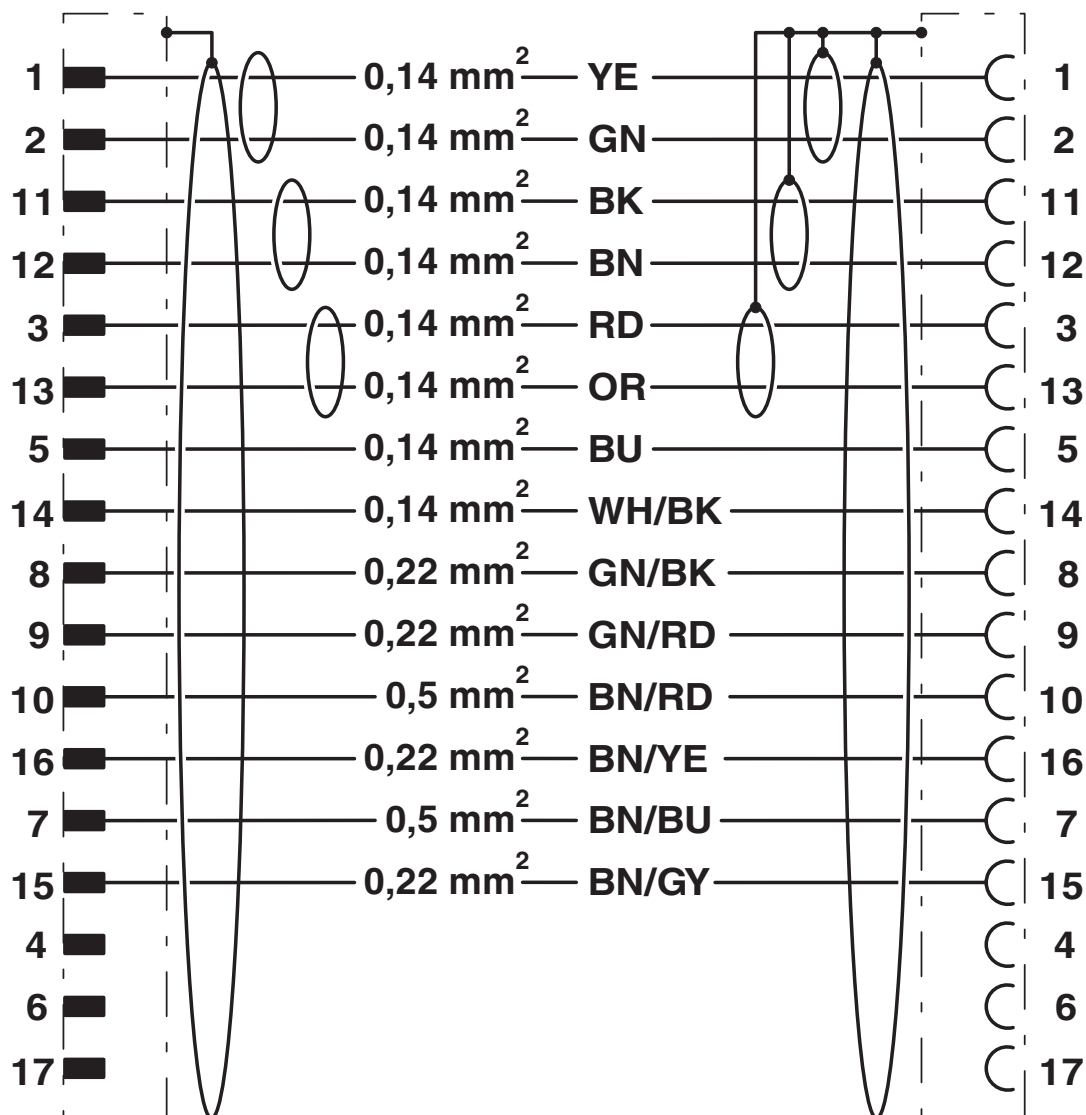
Diagrama eléctrico
