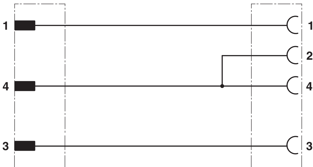
Ocupación de contactos de los conectores macho / hembra M12, puenteados
