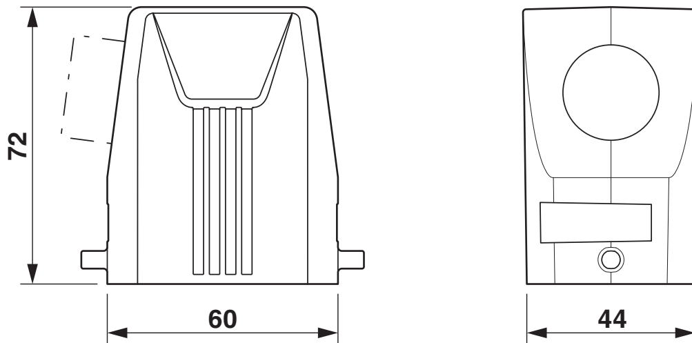
Maßzeichnung
