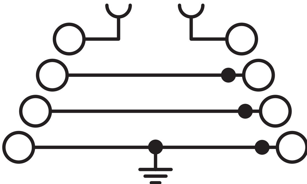
Schaltplan
