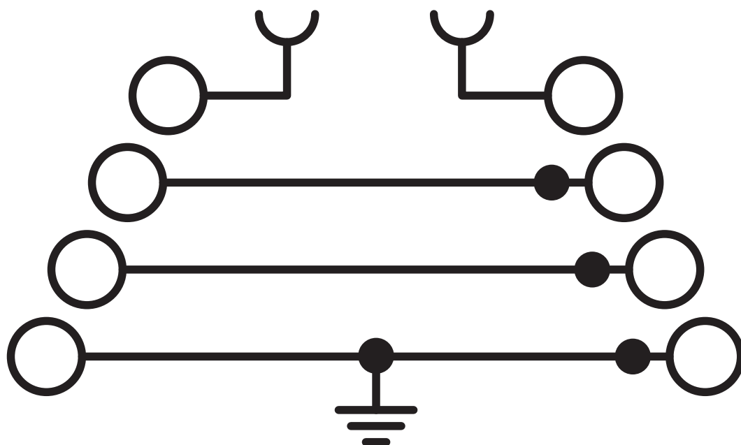
Diagrama eléctrico
