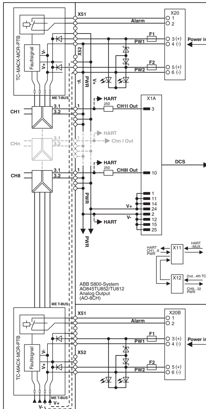
Blockschaltbild
