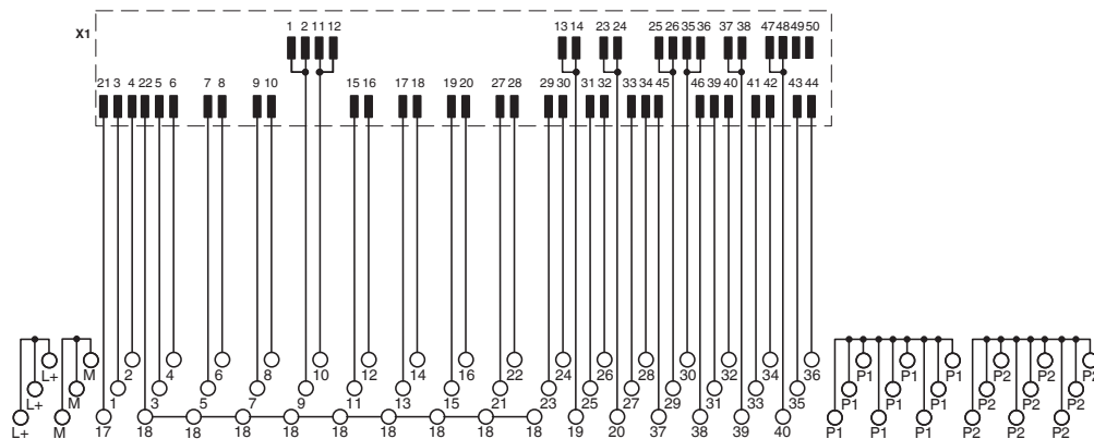
Schaltplan
