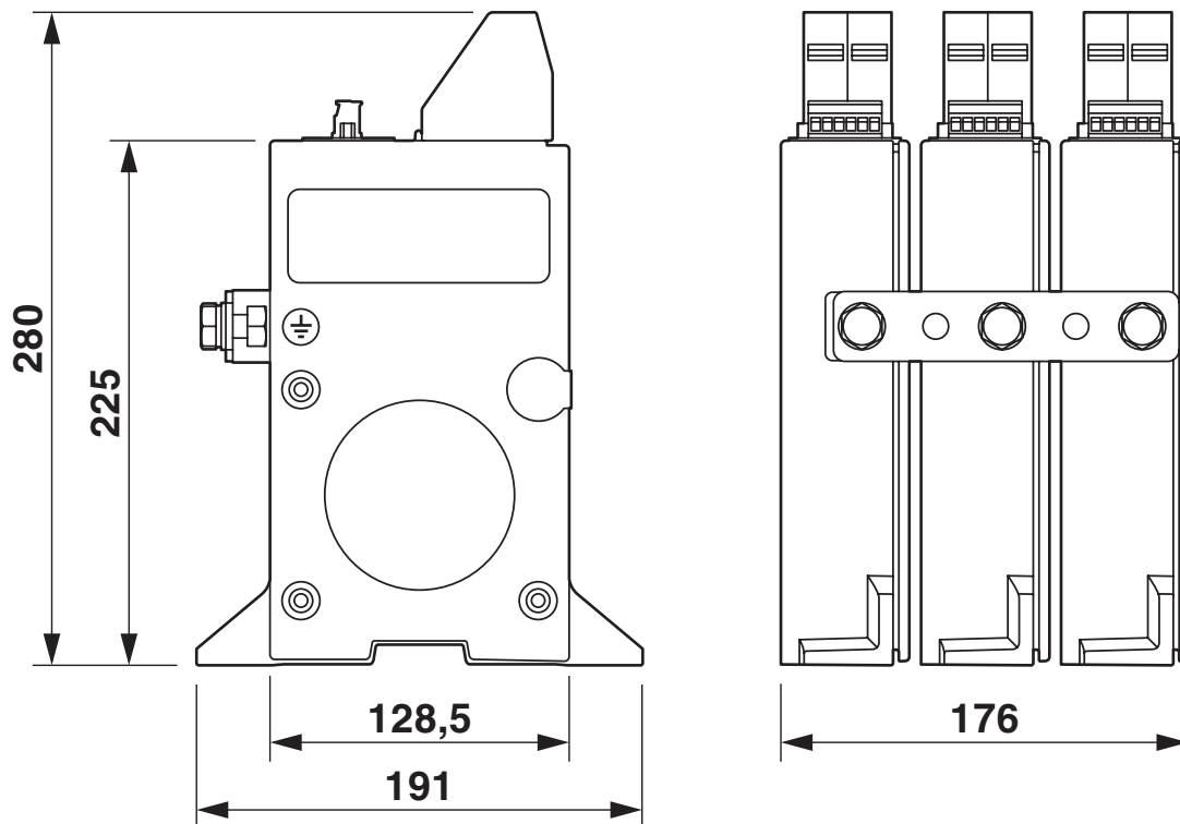
Maßzeichnung
