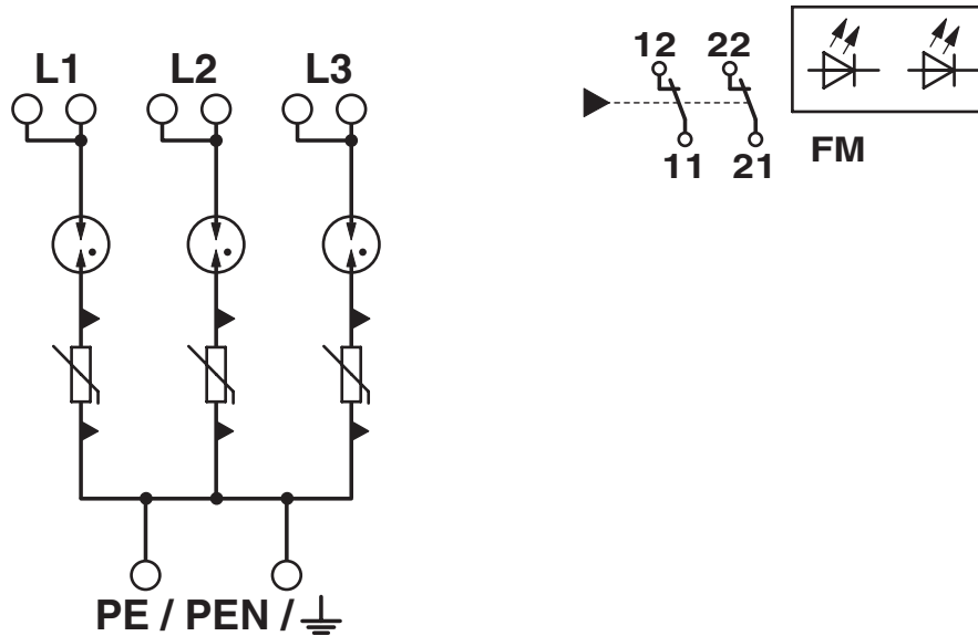
Schaltplan
