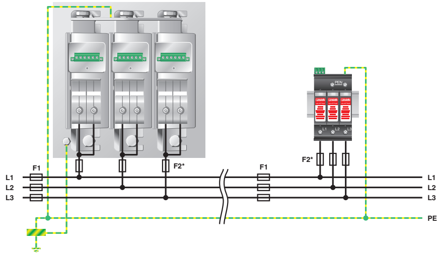
Applikationszeichnung
