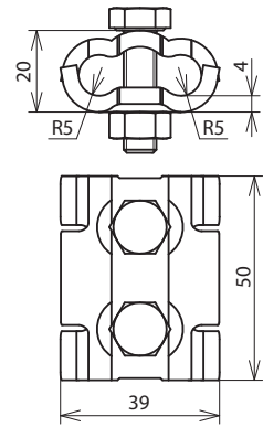
Maßbild PV 4.10 SKM8X30 CU
