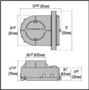
3111136 Boitier d'encastrement
