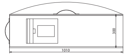
Maßbild KLT 101 30 10
