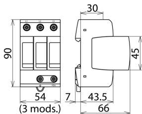
Dimensiones del DG M TNC 440
