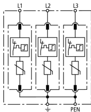
Esquema del DG M TNC 440
