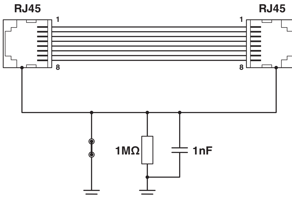
Diagrama eléctrico
