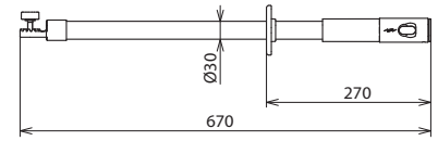
Maßbild IS ZK STK 670
