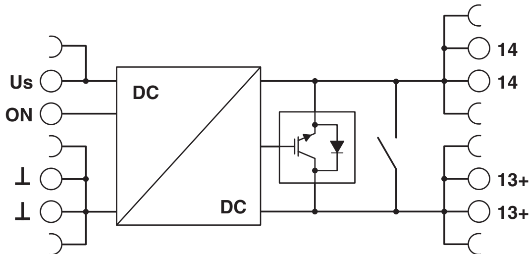
Schaltplan
