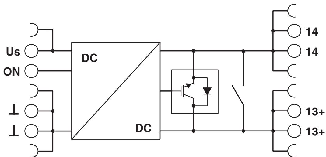
Diagrama eléctrico
