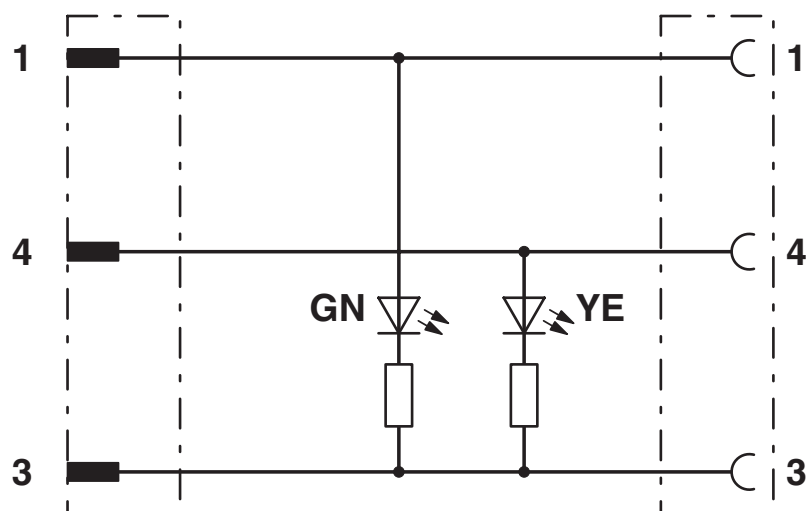
Diagrama eléctrico
