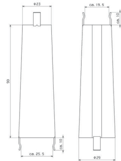
Maßbild PSS DII
