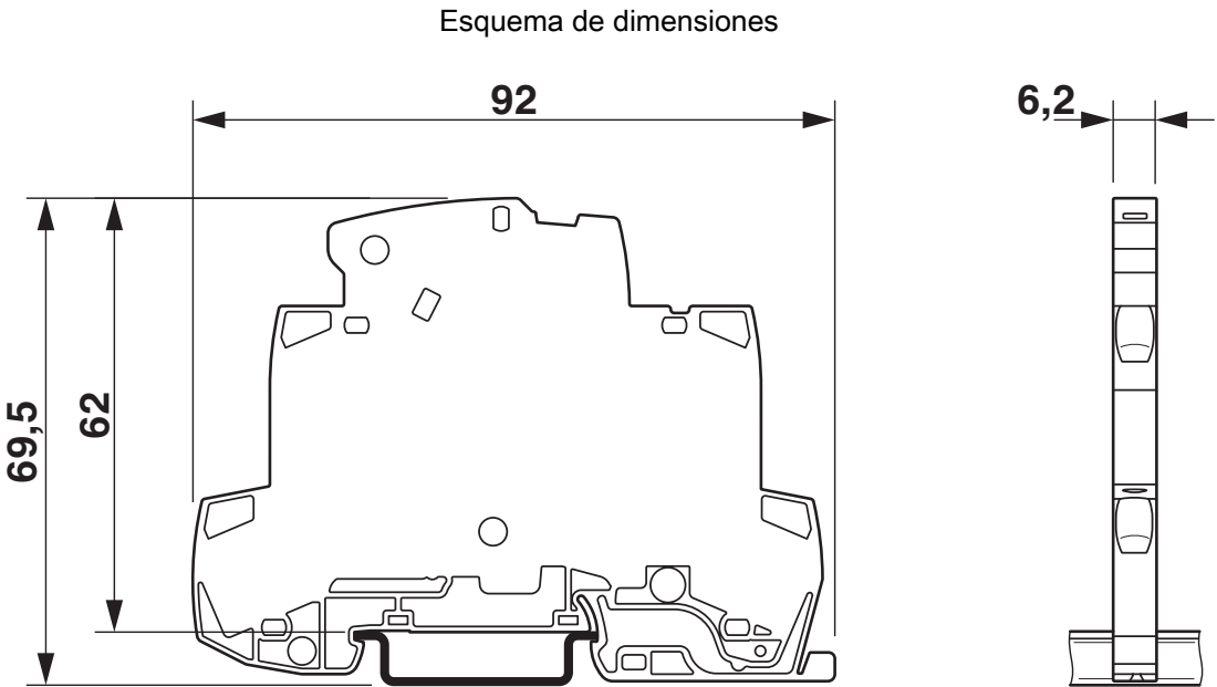
Plano esquemático
