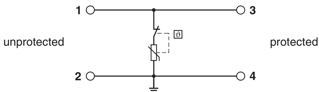
Diagrama eléctrico
