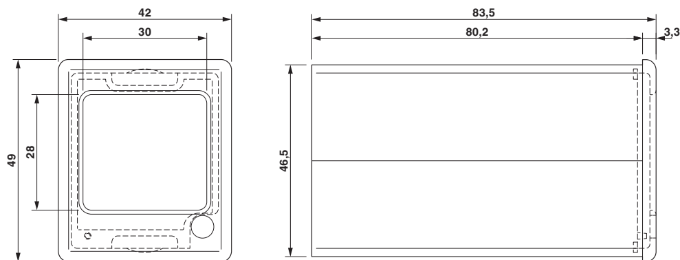
Esquema de dimensiones
