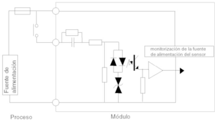
Diagrama del circuito de entrada
