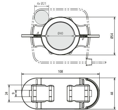
Maßbild BFS SR D40 4AE HVI LI PL KST
