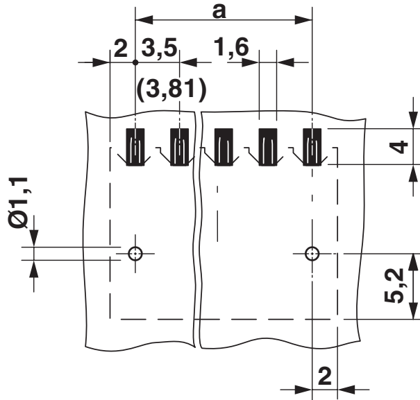
Bohrplan/Lötpadgeometrie
