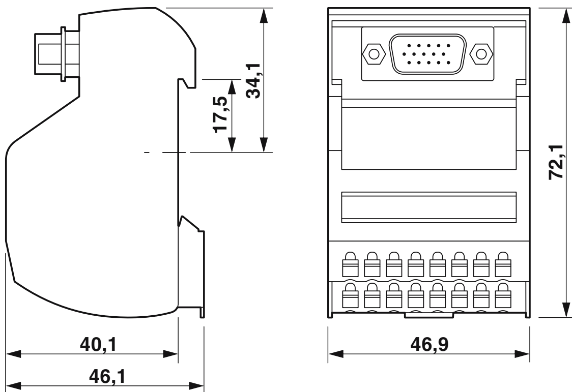
Maßzeichnung
