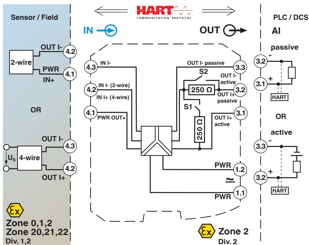
Schéma fonctionnel
