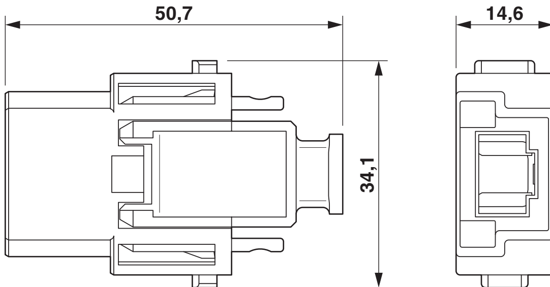
Maßzeichnung
