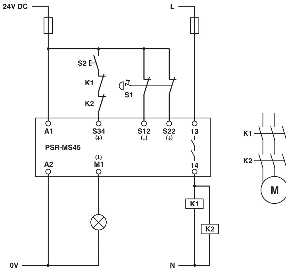
Diagrama eléctrico
