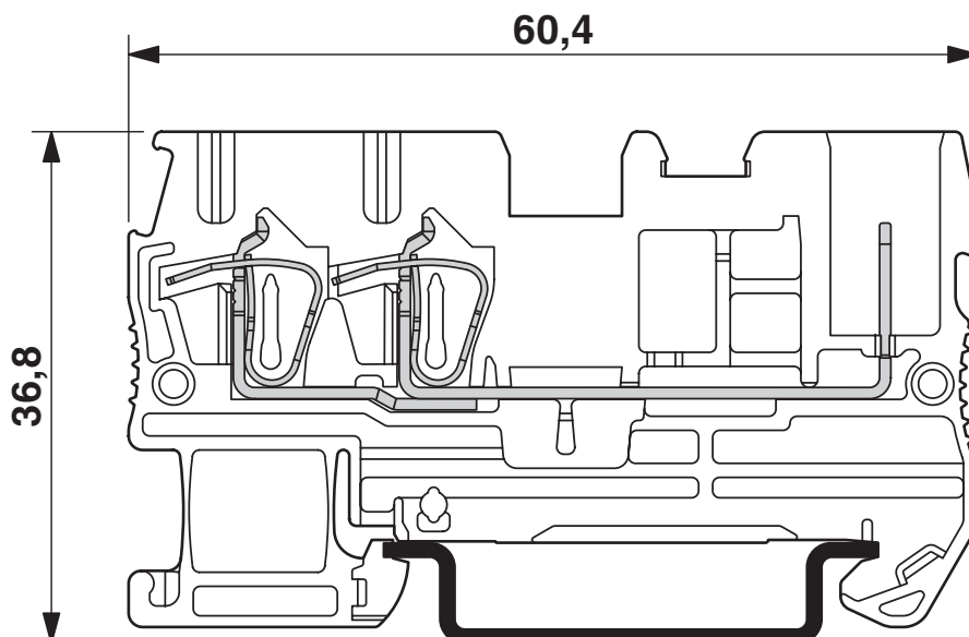
Dessin coté
