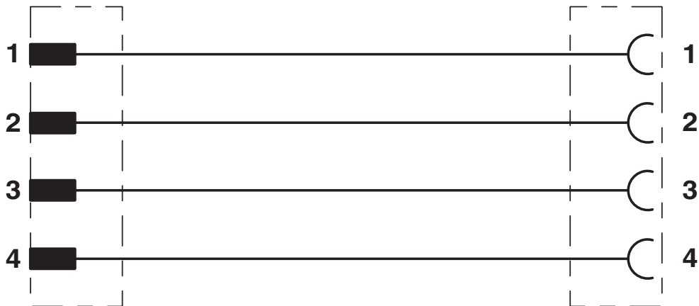
Diagrama eléctrico
