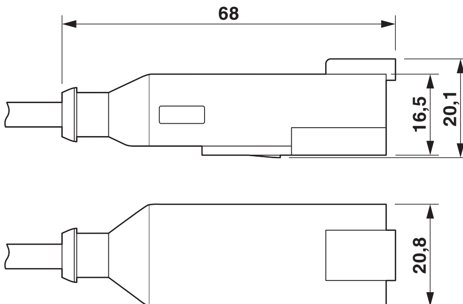
DEUTSCH DT04-4P, vista superior y lateral
