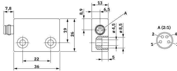
Maßzeichnung
