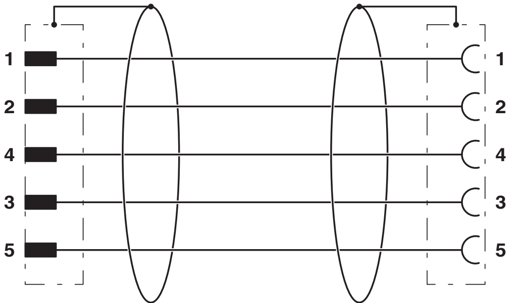
Schaltplan
