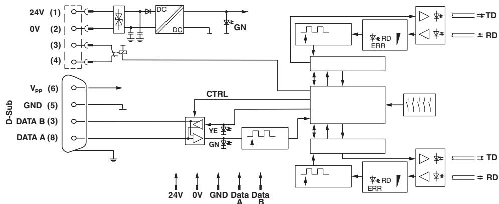
Schéma fonctionnel
