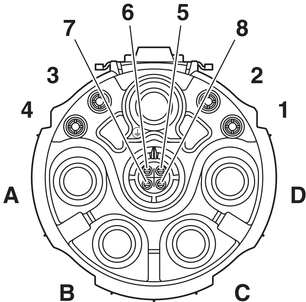
Schemazeichnung
