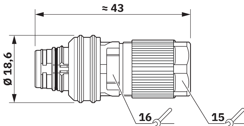
Maßzeichnung
