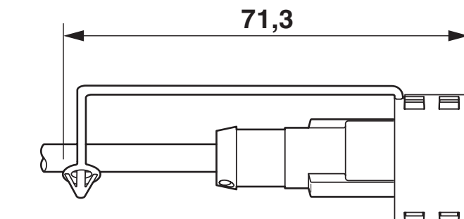
Maßzeichnung
