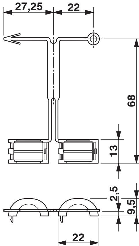
Dessin coté
