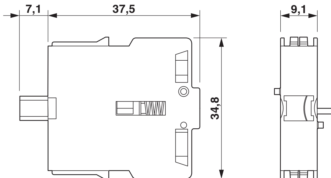
Dessin coté
