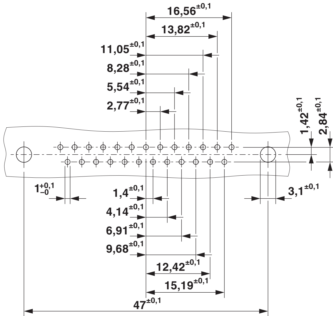
Bohrplan/Lötpadgeometrie
