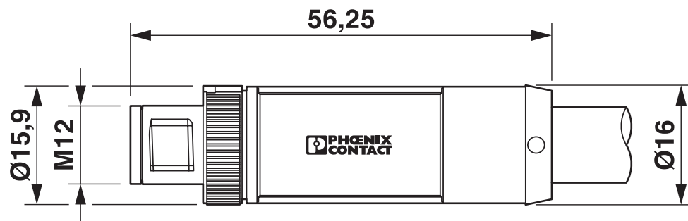
Maßzeichnung
