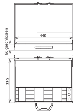
Maßbild SBKL EKS TI KVS 2F
