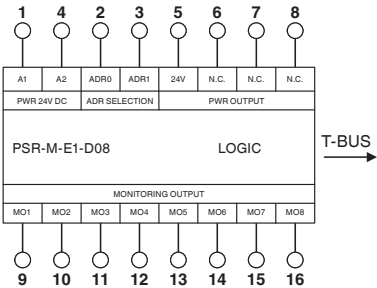
Blockschaltbild
